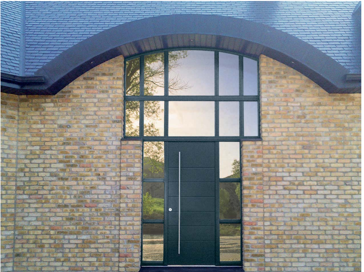
PHOSPHORE + FIXES EN DORMANT VITRÉS + IMPOSTE VITRÉE - COMPOSITION SUR MESURE - HAUTEUR TOTALE 3945 - LARGEURS : ENSEMBLE BAS 1800 - IMPOSTE 2470
